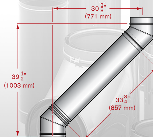
HE-10DE45-FD - 2 x Coude 45° HC-10DL3-FD - Longueur 36" (914 mm)
